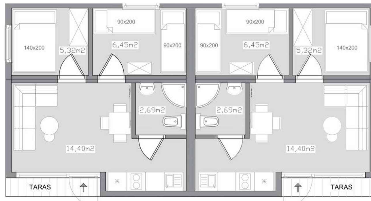
RZUT BUDYNKU M.3.1
