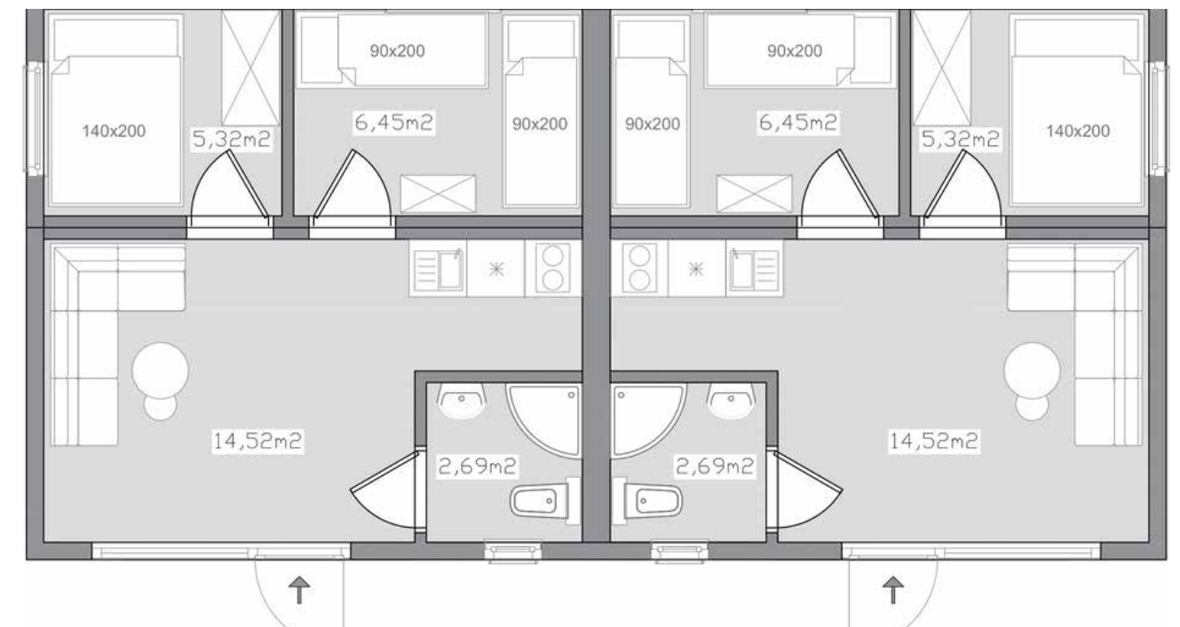
RZUT BUDYNKU M.3.2
